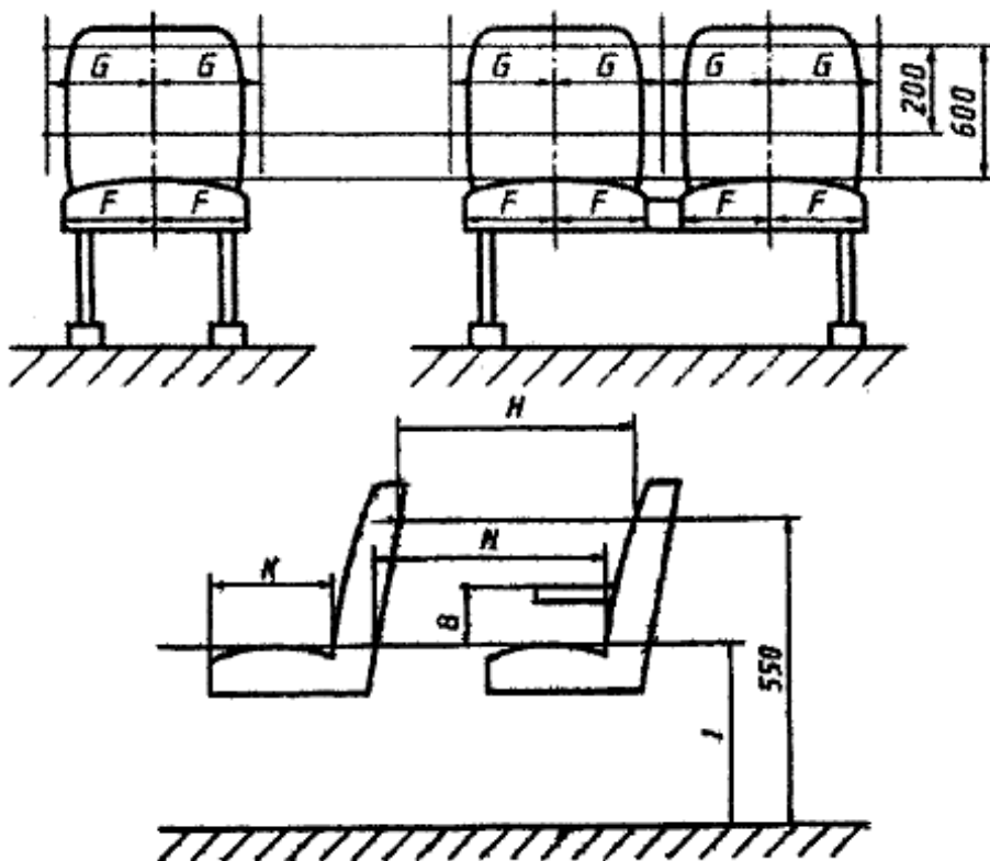
Рисунок 1.16.1. Размеры и расположение сидений
